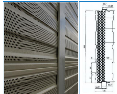
Nouveaux panneaux opaques plus épais et plus absorbants à installer
